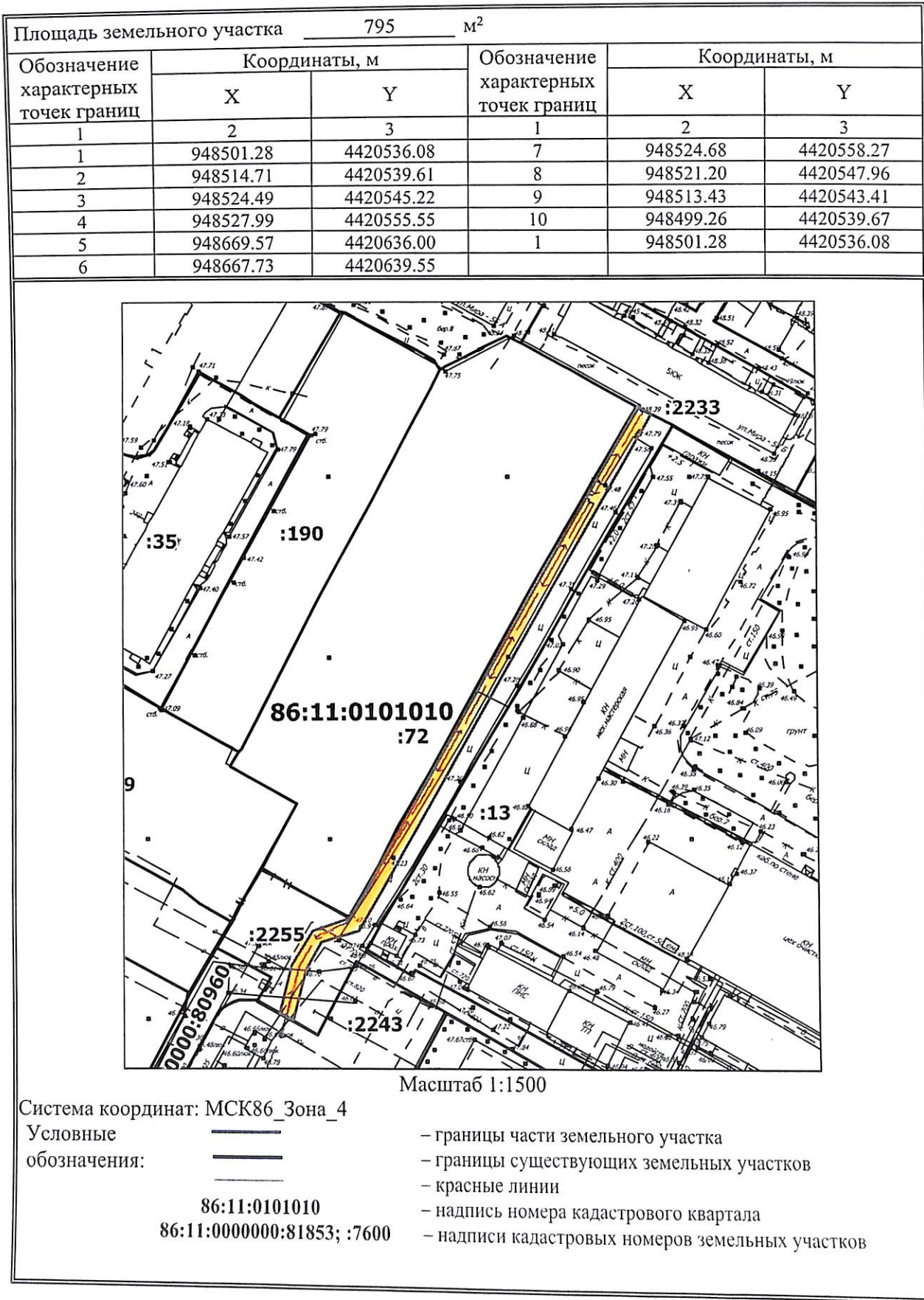
Схема границ сервитута на кадастровом плане территории
